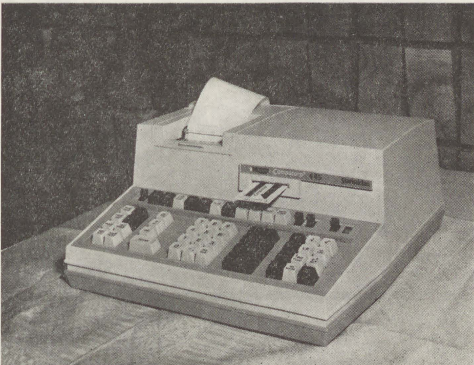
„CompuCorp 445 Statistician” asztali számítógép, a sorozat legnagyobb modellje, statisztikai számítások elvégzésére különösen alkalmas.
